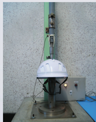
耐貫通性試験 厚生労働省保護帽規格による
